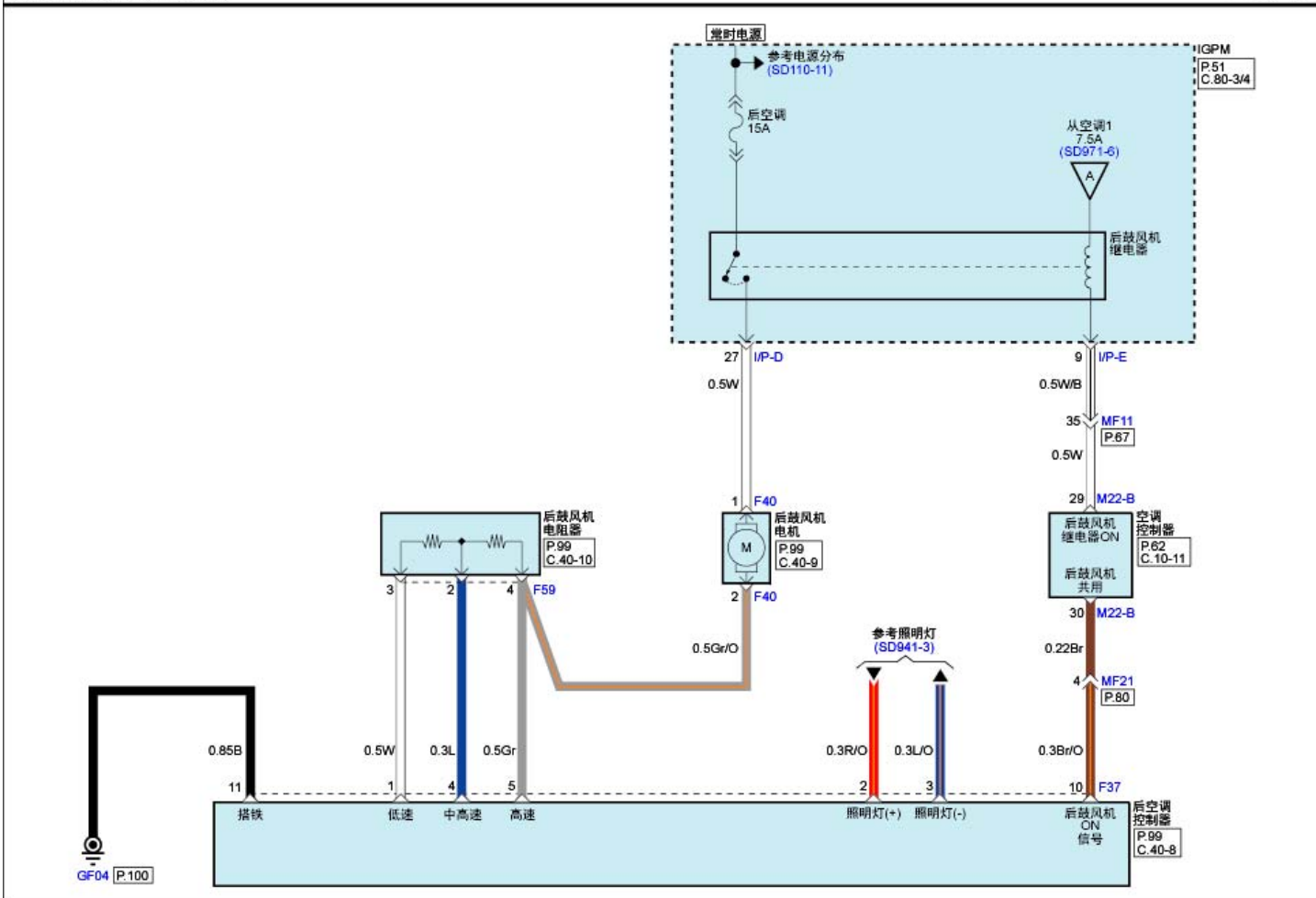
空调控制系统(手动)(4)
